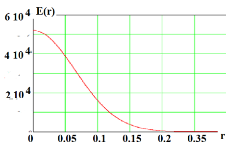
1-сурет. Диаметрі D=2,05 м параболоидты концентратордың фокусында ағын тығыздығының таралуы
